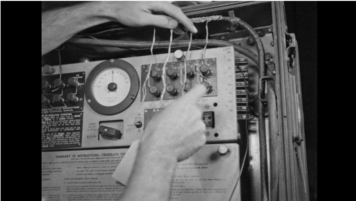
9. <TRANSFER OF 8TH ARMY COMCENTER, SEOUL TO YONGSAN, KOREA>(National Archives II, 111-LC-34117 / 미국 NA II 소장 노획영상 컬렉션 (4)) - 1953년 8월, 용산기지 캠프 코이너(Camp Coiner) 통신센터에서 반송파 통신장비의 전파 송수신 단자를 연결하고 있는 미군의 모습.
